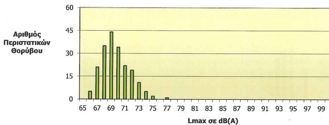
Κατανομή Στάθμης Θορύβου L_{max} Σταθμός: Ραφήνα (NMT 7) Συνολικός Αριθμός Συσχετισμένων Περιστατικών Θορύβου: 199
