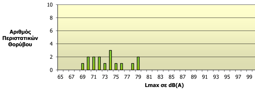
Κατανομή Στάθμης Θορύβου Lmax Σταθμός: Σπάτα (NMT 10) Συνολικός Αριθμός Συσχετισμένων Περιστατικών Θορύβου: 16
