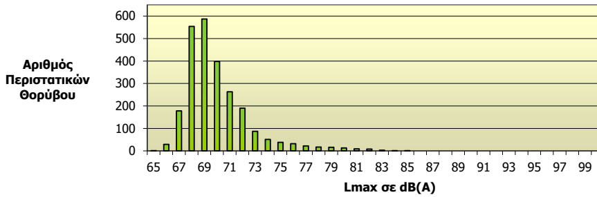
Κατανομή Στάθμης Θορύβου Lmax Σταθμός: Κορωπί (NMT 9) Συνολικός Αριθμός Συσχετισμένων Περιστατικών Θορύβου: 2498
