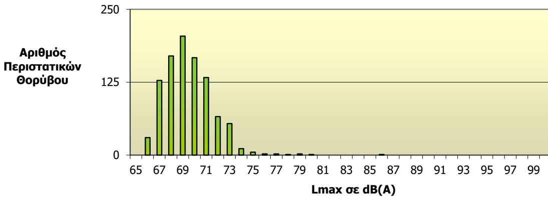
Κατανομή Στάθμης Θορύβου L max Σταθμός: Ραφήνα (NMT 7) Συνολικός Αριθμός Συσχετισμένων Περιστατικών Θορύβου: 977
