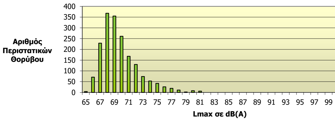
Κατανομή Στάθμης Θορύβου L max Σταθμός: Κορωπί (NMT 9) Συνολικός Αριθμός Συσχετισμένων Περιστατικών Θορύβου: 1827
