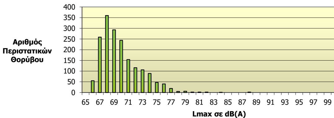
Κατανομή Στάθμης Θορύβου L max Σταθμός: Κορωπί (NMT 9) Συνολικός Αριθμός Συσχετισμένων Περιστατικών Θορύβου: 1802
