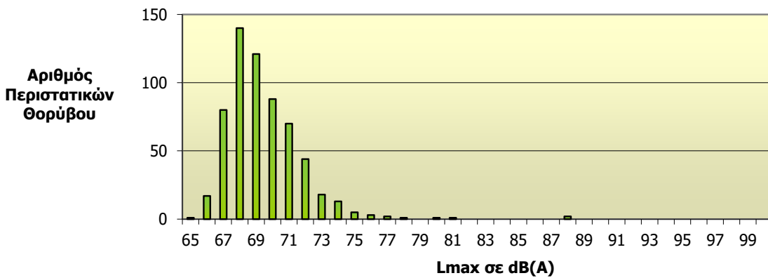
Κατανομή Στάθμης Θορύβου L_{max} Σταθμός: Ραφήνα (NMT 7) Συνολικός Αριθμός Συσχετισμένων Περιστατικών Θορύβου: 607
