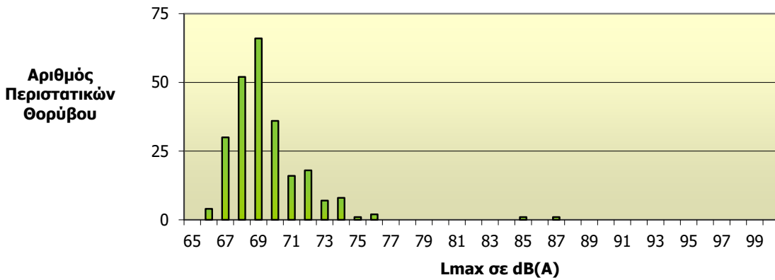
Κατανομή Στάθμης Θορύβου L_{max} Σταθμός: Άγιος Νικόλαος (NMT 6) Συνολικός Αριθμός Συσχετισμένων Περιστατικών Θορύβου: 242
